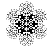
6x36(WS)+IWRC
