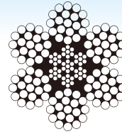
6x19+IWRC
