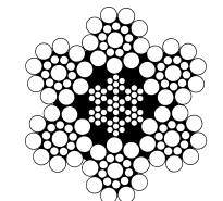
6x19(S)+IWRC
