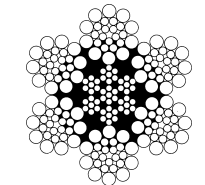
6x26(WS)+IWRC
