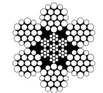
6x19(W)+IWRC
