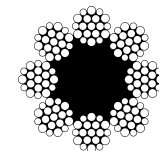
8 x 19 (W)+FC
